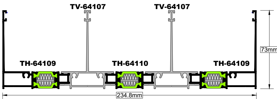
Πλευρικός και Άνω Τετράφυλλος Οδηγός Επαλλήλου 73mm / Side and Upper Quadruple Successive Rail Sash 73mm
