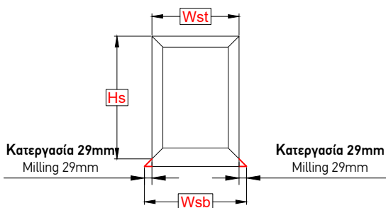
Υπόδειγμα Φύλλου Τζαμιού Glass Sash Model
