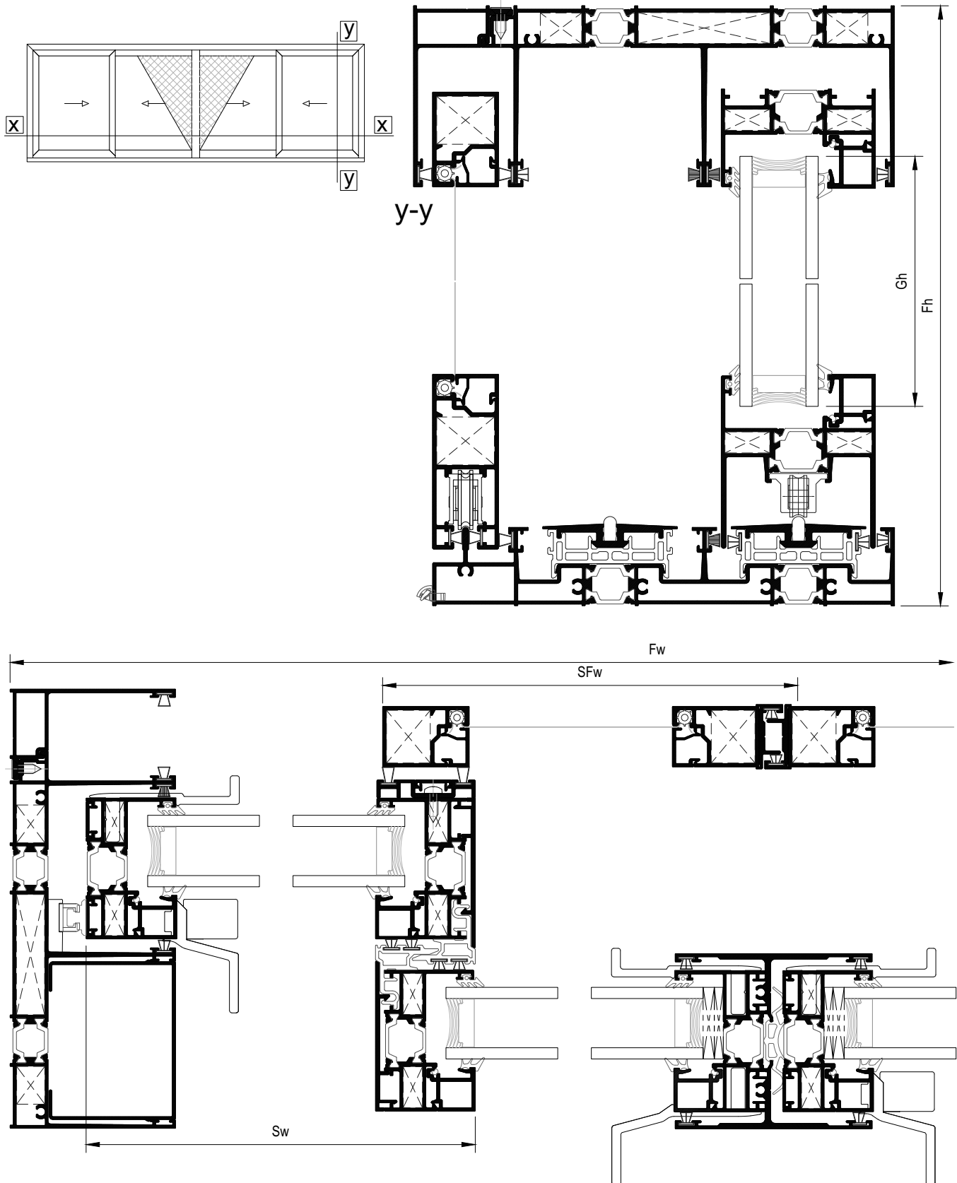
Cf Four-sash meeting stile sliding window with flyscreen Τετράφυλλο φιλητό συρόμενο με σήτα
