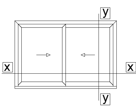
A Two-sash sliding window Δίφυλλο επάλληλο συρόμενο
